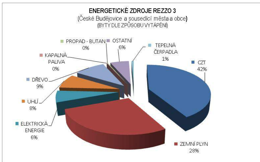
GRAF ČÍSLO 8: POČET BYTŮ DLE ZPŮSOBU VYTÁPĚNÍ V ČESKÝCH BUDĚJOVICÍCH A V SOUSEDÍCÍCH MĚSTECH A OBCÍCH (REZZO 3)
