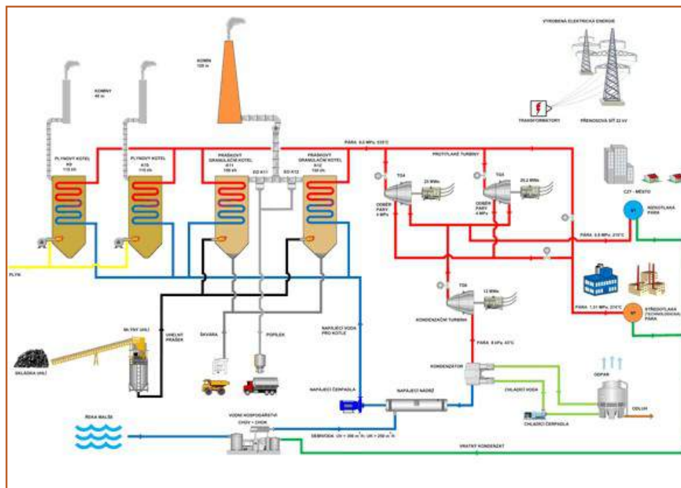
OBRÁZEK ČÍSLO 72: SCHÉMA ZAPOJENÍ
