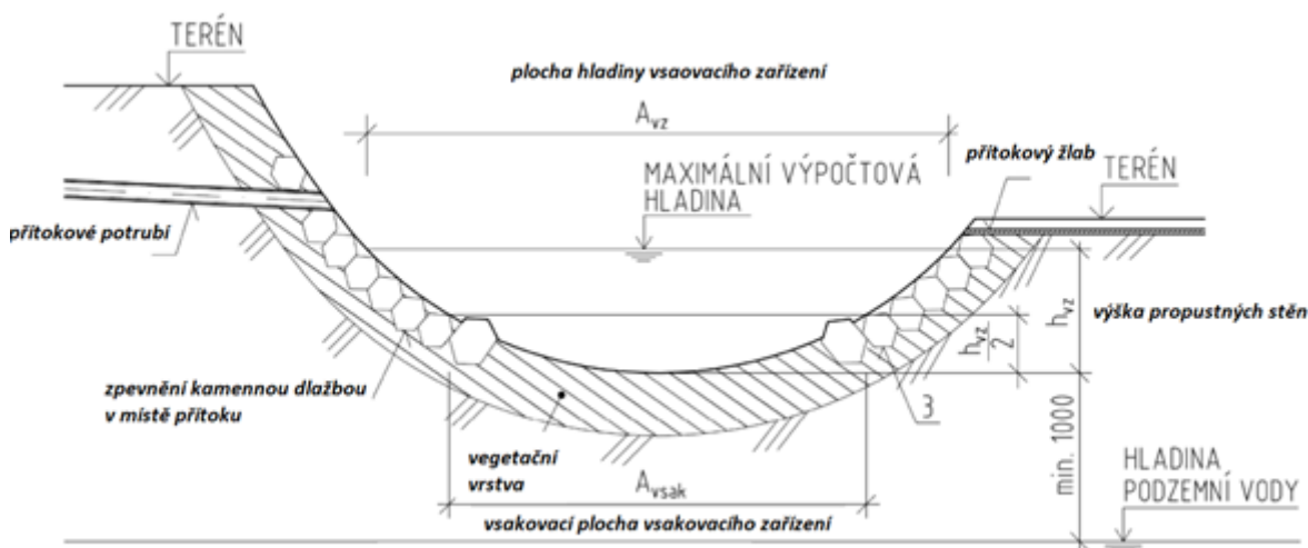
Obrázek: Vsakovací rýha (zdroj: Vsakování srážkových vod, Metodická pomůcka MMR, 2019, upraveno)
