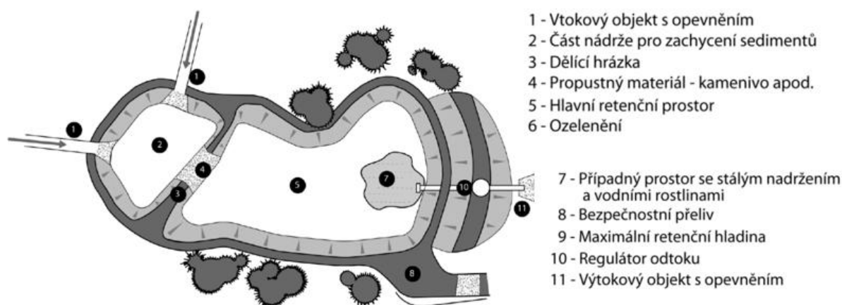
Obrázek: Povrchová suchá vsakovací nádrž
